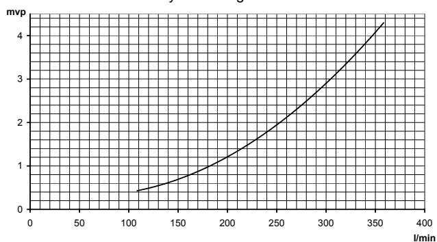
Tryckfallsdiagram
